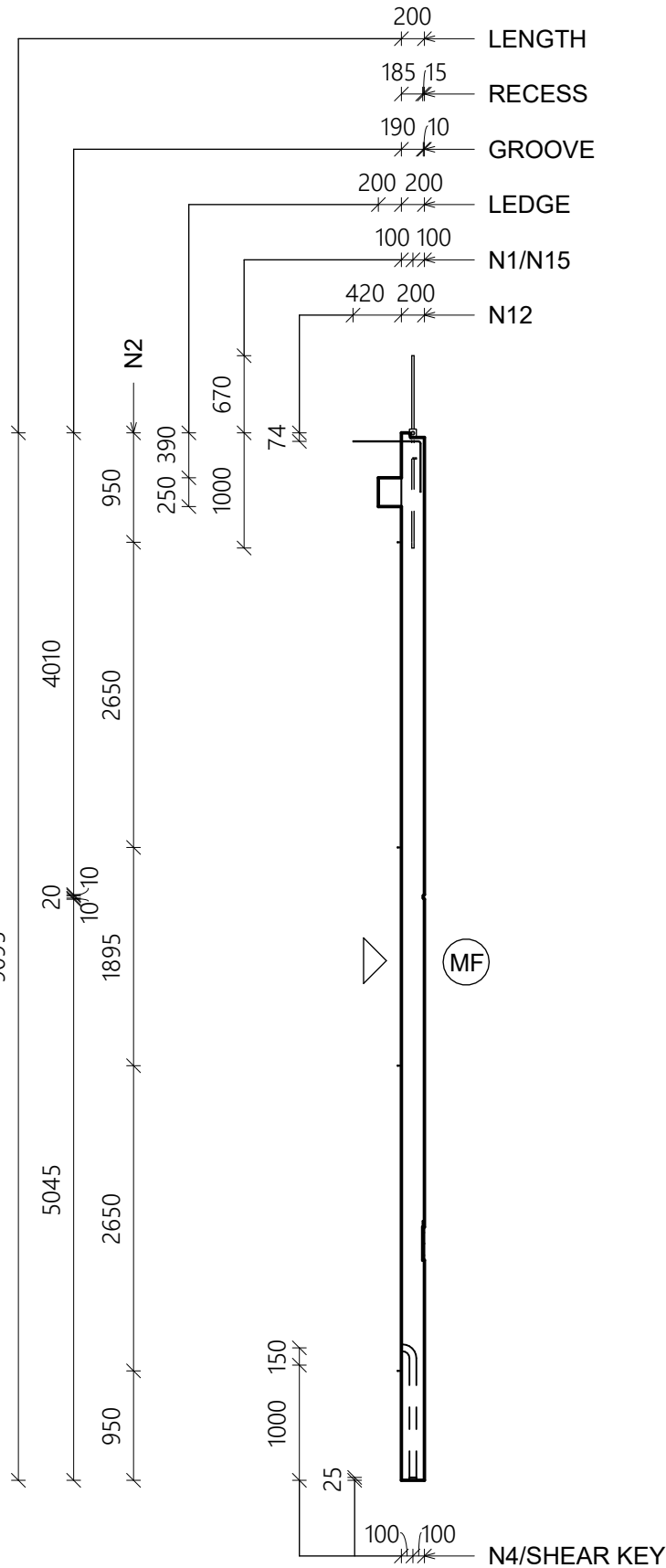
1 SECTION 1 : 60
