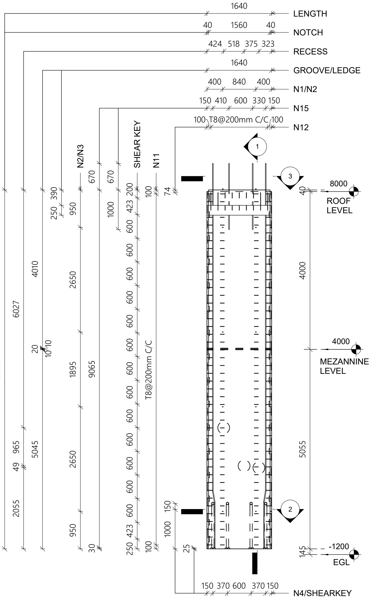
A ELEVATION 1 : 60
