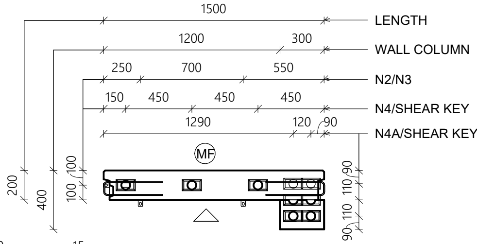
SECTION 4 1 : 25
