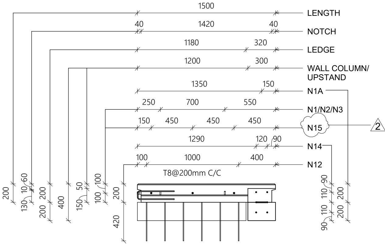
SECTION 3 1 : 25
