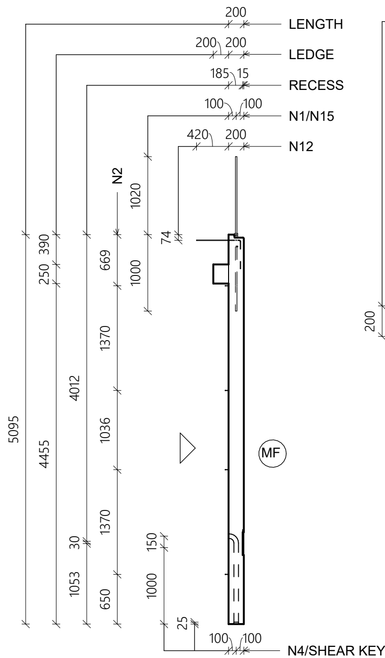
SECTION 2 1 : 50
