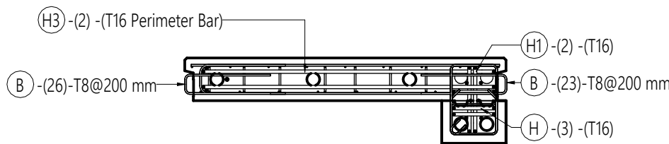
5 SECTION (REINF) 1 : 25
