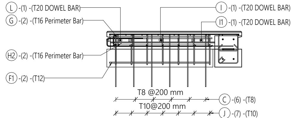
3 SECTION (REINF) 1 : 25
