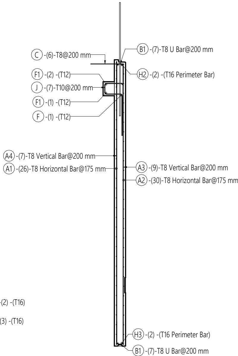
2 SECTION (REINF) 1 : 40
