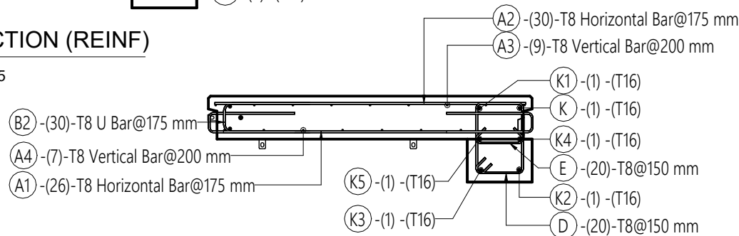
4 SECTION (REINF) 1 : 25
