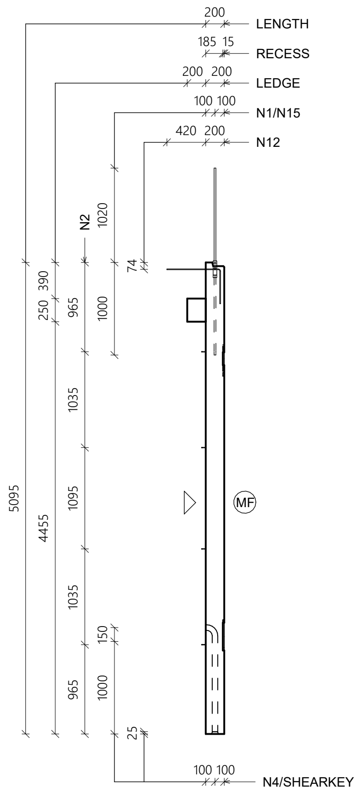
1 SECTION 1 : 40
