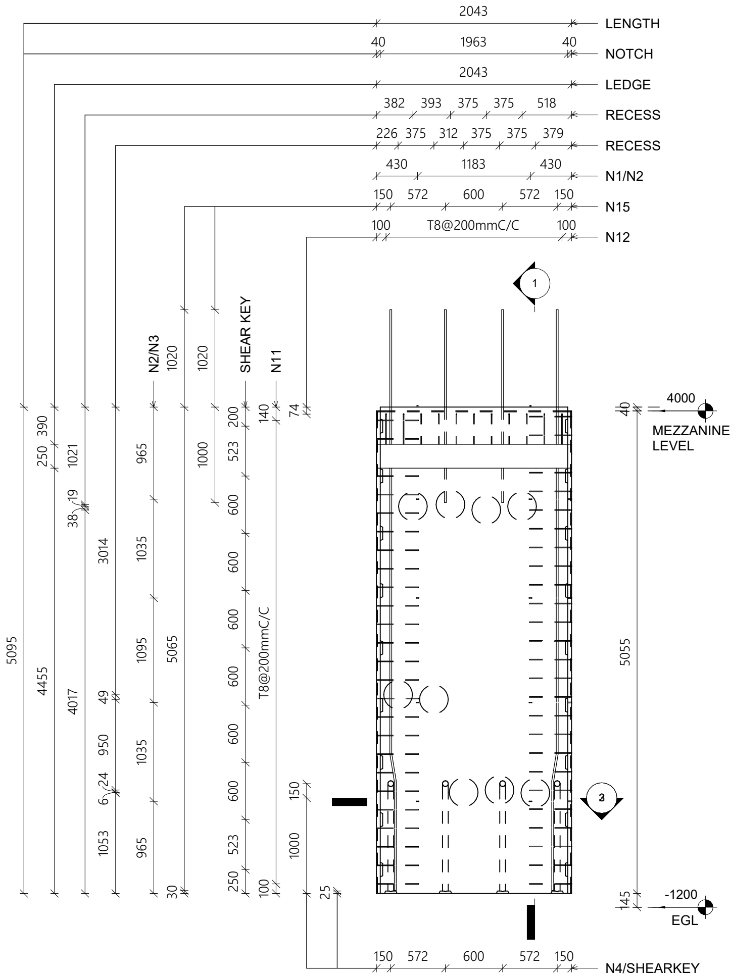
A ELEVATION 1 : 40
