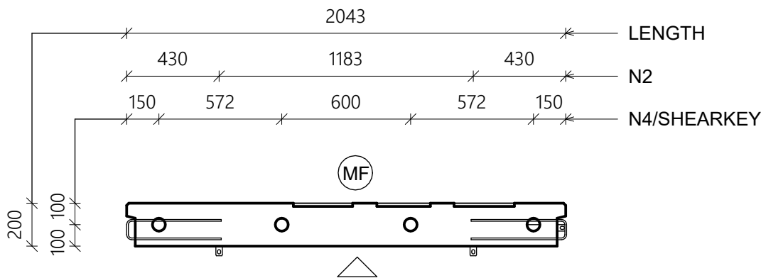
SECTION 3 1 : 25
