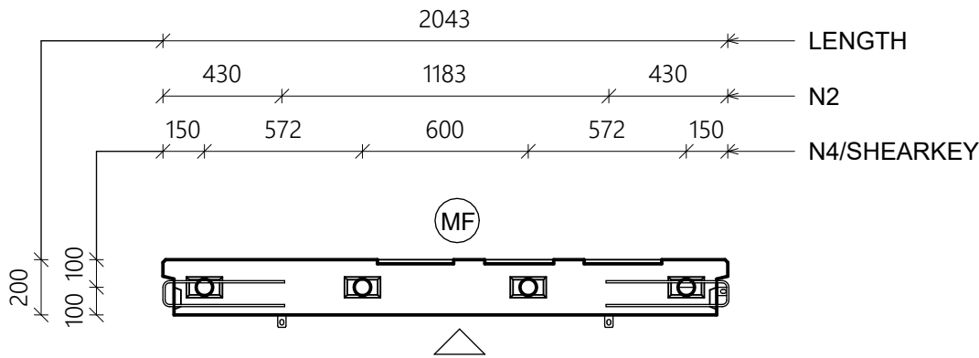
SECTION 2 1 : 25
