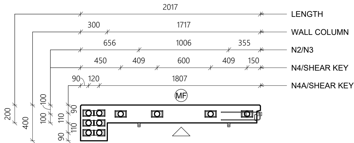
3 SECTION 1 : 25
