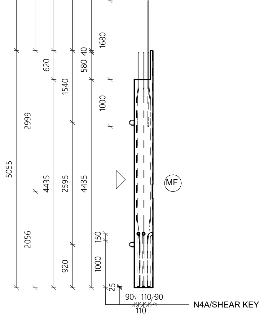
2 SECTION 1 : 50
