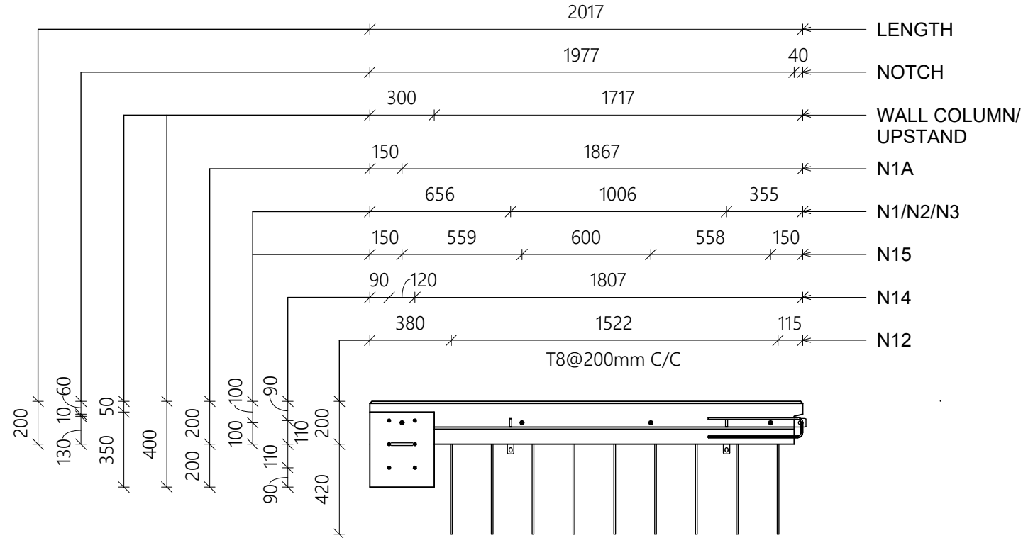
3 SECTION 1 : 25
