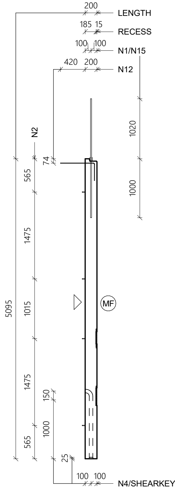
SECTION 1 : 40
