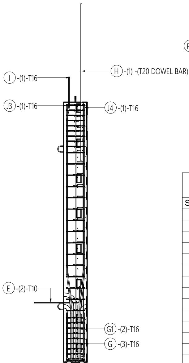
2 SECTION (REINF) 1 : 40
