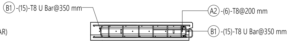
5 SECTION (REINF) 1 : 25
