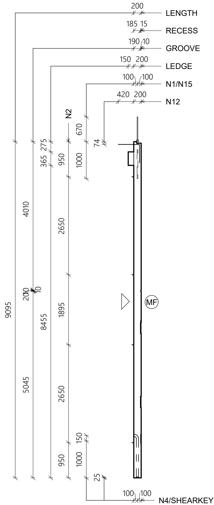
1 SECTION 1 : 60
