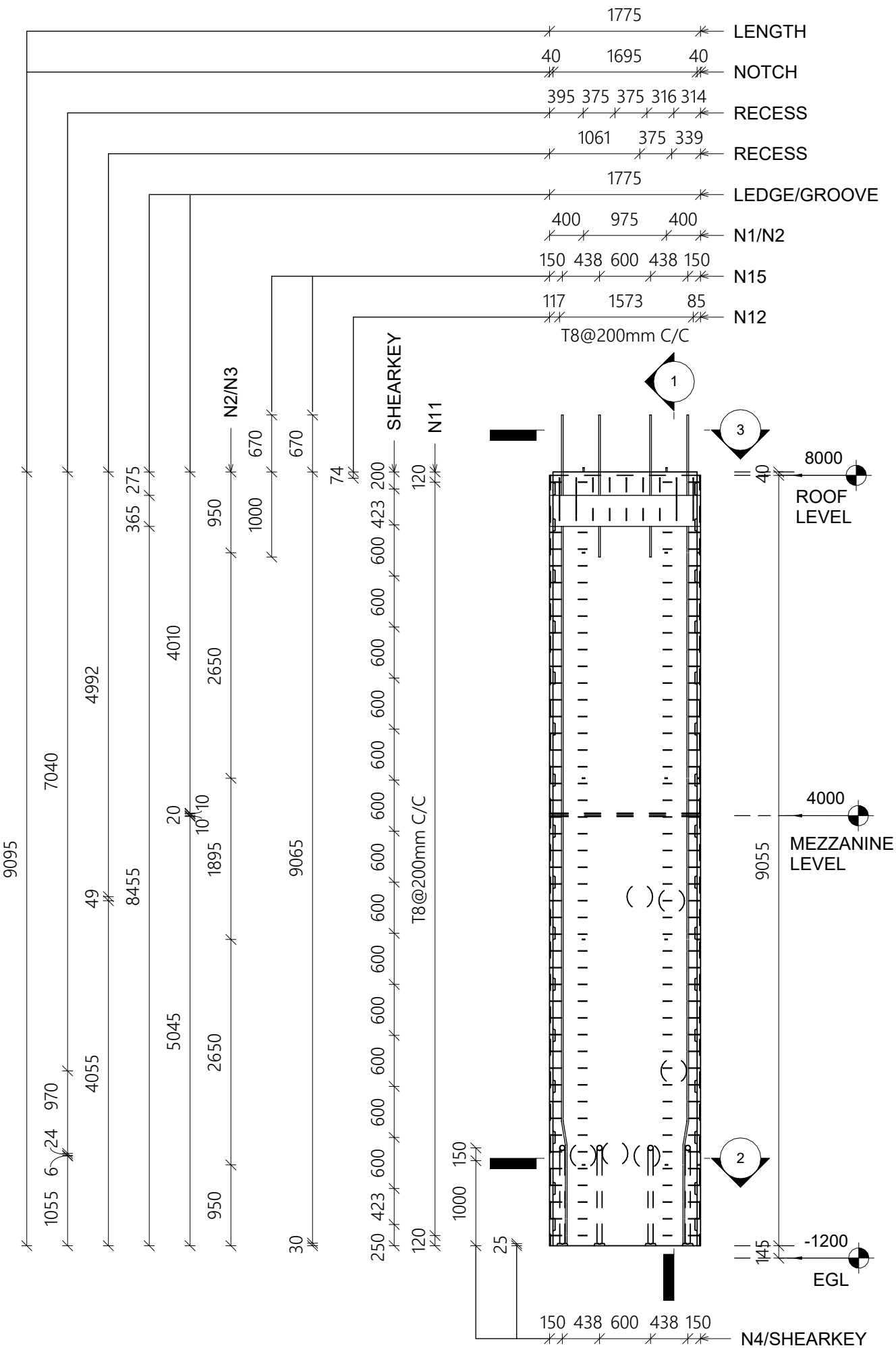
A ELEVATION 1 : 60
