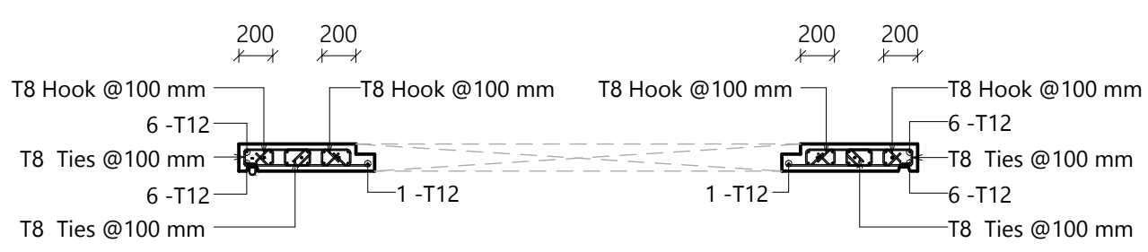
4 SECTION(REINF) 1 : 40
