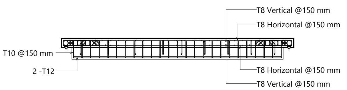
3 SECTION(REINF) 1 : 40
