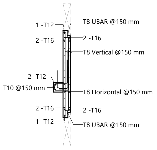
2 SECTION(REINF) 1 : 40
