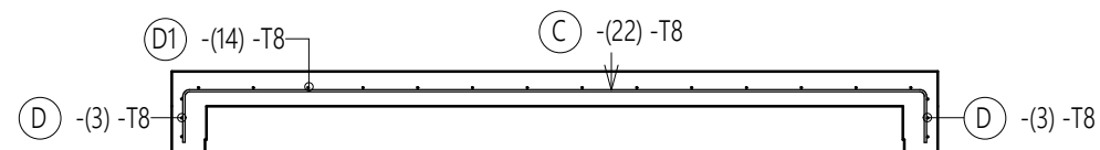
2 SECTION REINF 1 : 30
