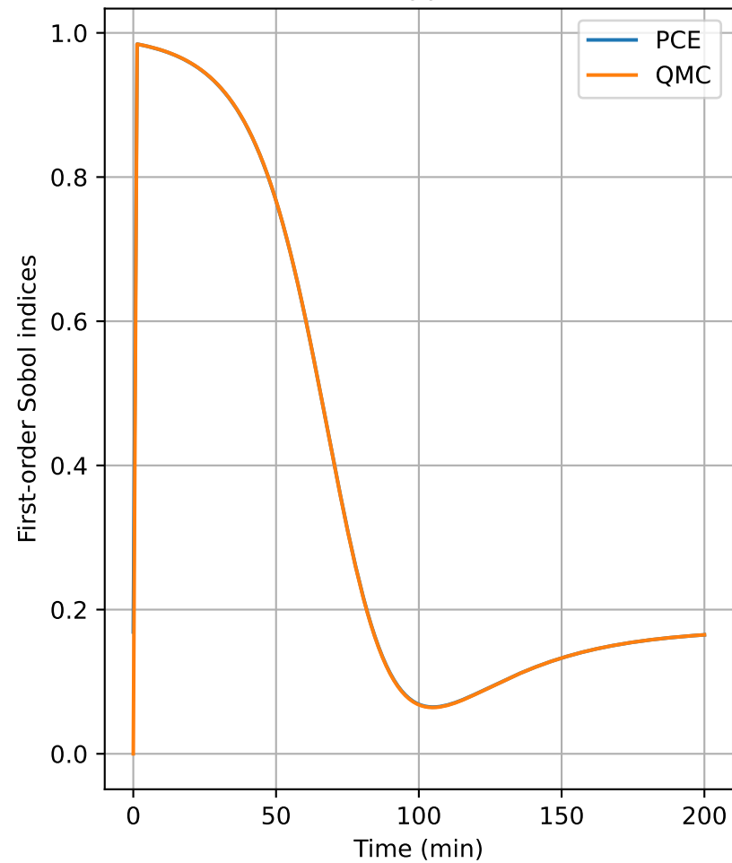
kappa
