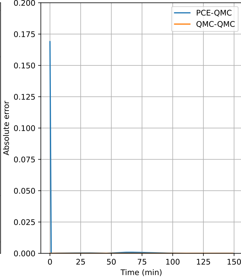
Sobol index error (Absolute)
