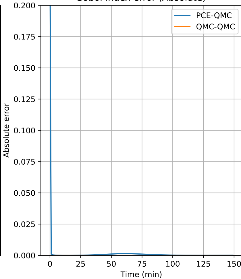
Sobol index error (Absolute)
