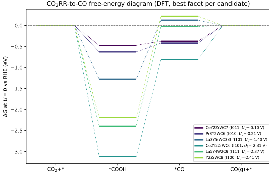
Figure 4.7: 여섯 후보의 CO 2 → CO 전산 수소 전극(CHE) 자유에너지 다이어그램( U = 0 vs RHE, 후보별 최적 면). 낮은 과전위 후보(CeY 2 ZrWC 7 , Pr 3 Y 2 WC 6 )는 *COOH가 온전한 중간 상태인 반면, 나머지는 *COOH 심우물로 두 번째 환원이 강하게 흡열이다.
