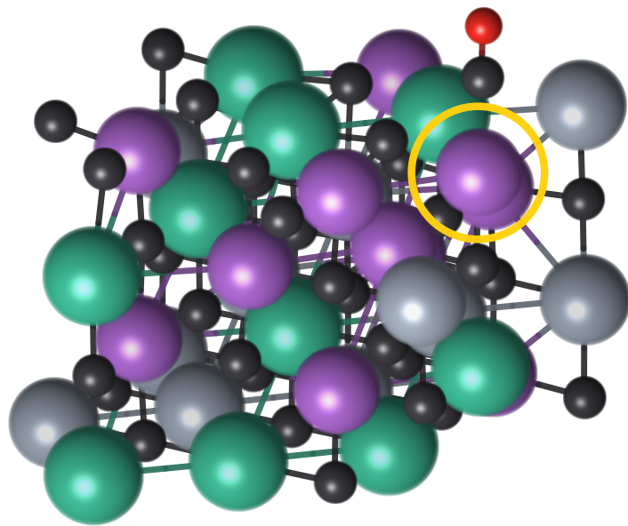
(a) (Mo, Ti, Zr)C
