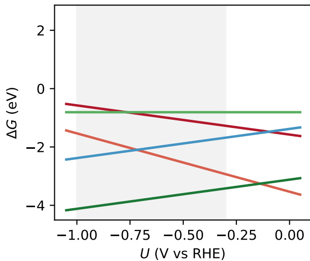
La5Y4W2C9 (facet 111)
