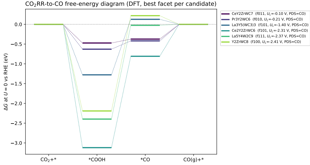
Figure 4.7: 여섯 후보의 CO 2 → CO 전산 수소 전극(CHE) 자유에너지 다이어그램 ( U = 0 vs RHE, 후보별 최적 면). 낮은 과전위 후보(CeY 2 ZrWC 7 , Pr 3 Y 2 WC 6 )는 *COOH가 온건한 중간 상태인 반면, 나머지는 *COOH 심우물로 두 번째 환원이 강하게 흡열이다.
