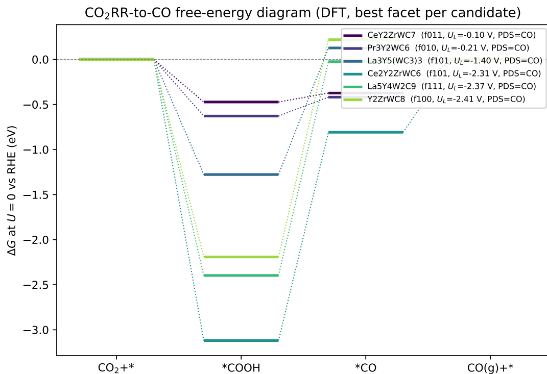
Figure 4.7: 여섯 후보의 \text{CO}_2 \rightarrow \text{CO} 전산 수소 전극(CHE) 자유에너지 다이어그램( U = 0 vs RHE, 후보별 최적 면). 낮은 과전위 후보( \text{CeY}_2\text{ZrWC}_7 , \text{Pr}_3\text{Y}_2\text{WC}_6 )는 \text{*COOH} 가 온건한 중간 상태인 반면, 나머지는 \text{*COOH} 심우물로 두 번째 환원이 강하게 흡열이다.
