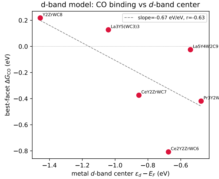
Figure 4.8: 금속 d -밴드 중심 \varepsilon_d - E_F 대 최적 면 \Delta G_{CO}^* . d -밴드가 높을수록 CO 결합이 강해지는 경향(추세선)으로 전도 특성과 흡착을 연결한다.
