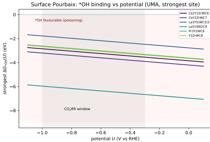
Figure 4.9: 표면 Pourbaix: 최강 결합 자리의 \Delta G_{*OH}(U) 대 전위(UMA). 작동창(음영) 전역에서 \Delta G_{*OH} < 0 이면 *OH 피복(산화/피독)이 예측된다.
