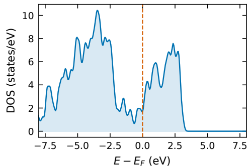
Y2ZrWC8 DOS( E_F )=1.7
