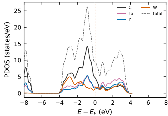
La5Y4W2C9
