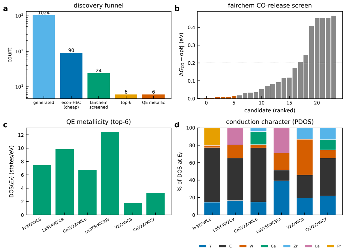
Figure 4.1: 종단간 발견 종합. (a) 1024개 생성 구조에서 6개 DFT 검증 금속성 후보까지의 발견 갈때기. (b) 스크리닝된 후보의 UMA 표면 일산화탄소 방출 디스크립터(상위 6개 강조). (c) 상위 6개의 페르미 준위 DFT 상태밀도. (d) 원소 투영 전도 특성 ( E_F 에서의 원소별 DOS 비중).
