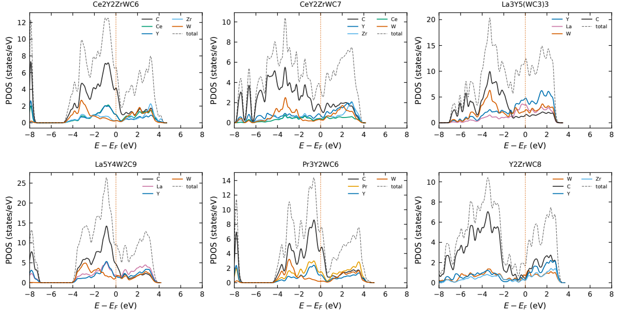
Figure 4.5: 여섯 DFT 검증 후보의 원소 투영 상태밀도(PDOS), E - E_F 기준. E_F (파선)에서의 유한 상태가 금속성을 확인하며, 원소별 분해가 전도 특성을 규명한다.
