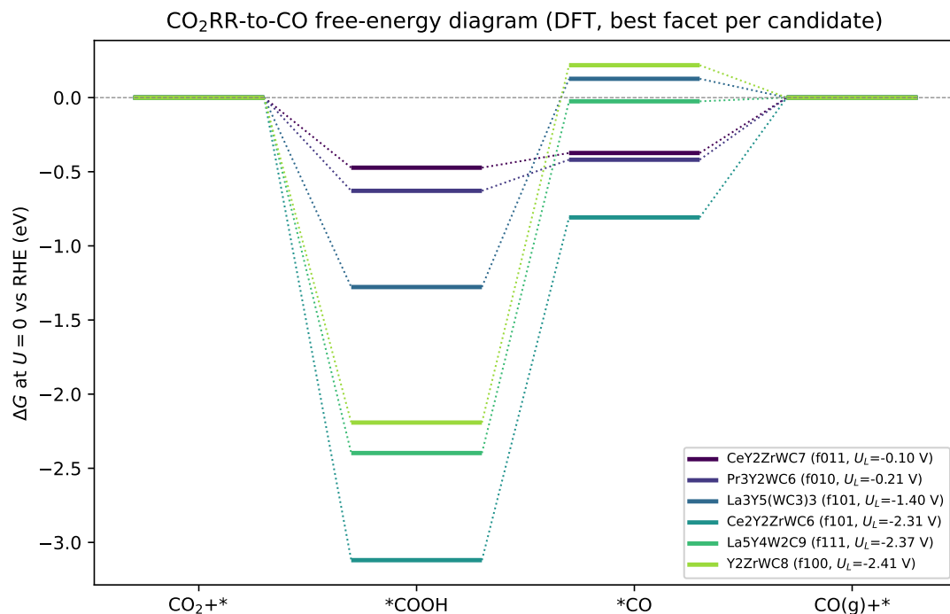
Figure 4.7: 여섯 후보의 CO 2 → CO 전산 수소 전극(CHE) 자유에너지 다이어그램( U = 0 vs RHE, 후보별 최적 면). 낮은 과전위 후보(CeY 2 ZrWC 7 , Pr 3 Y 2 WC 6 )는 *COOH가 온전한 중간 상태인 반면, 나머지는 *COOH 침우물로 두 번째 환원이 강하게 흡열이다.
