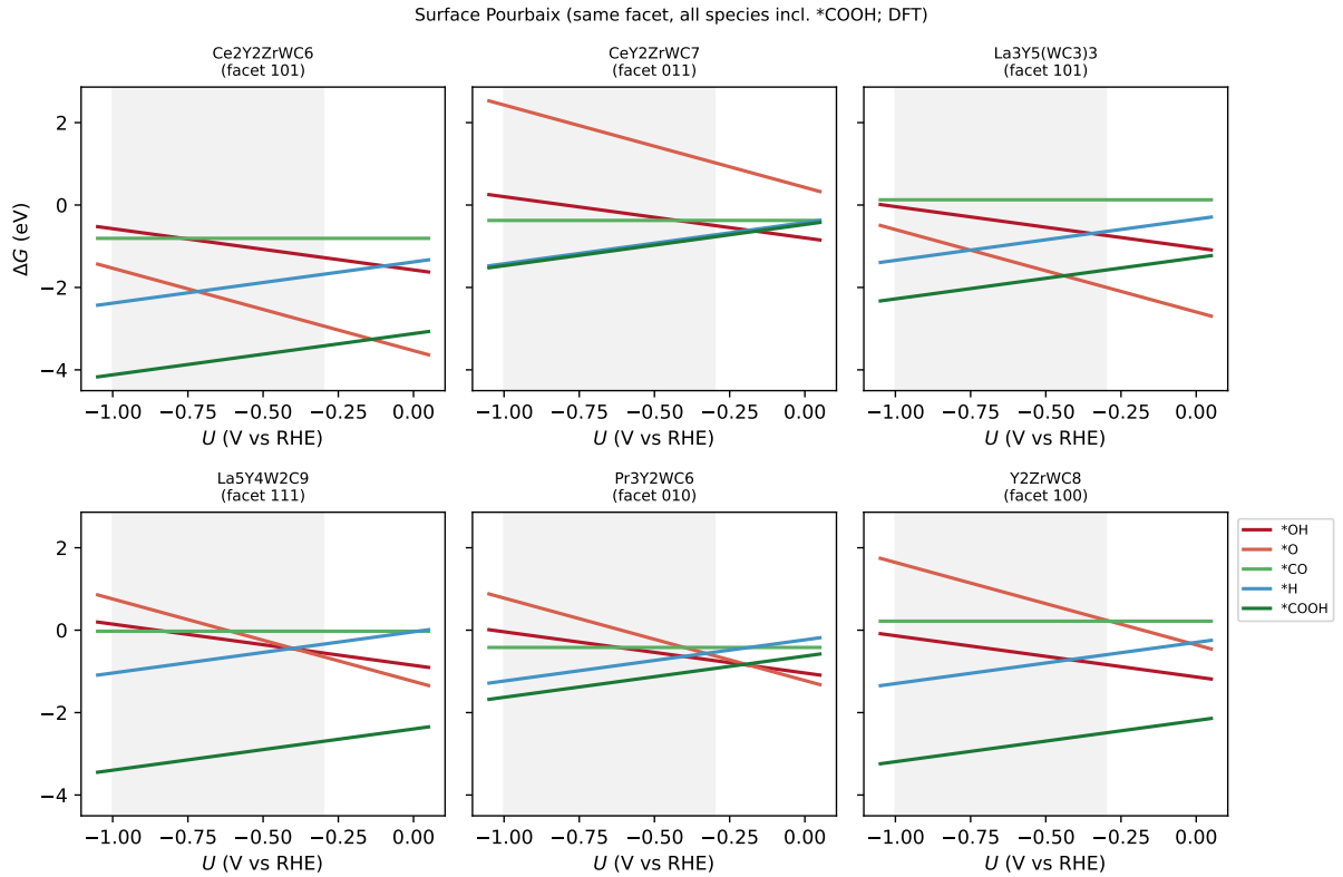
Figure 4.9: 여섯 후보의 활성 면 같은-면 완전 표면 Pourbaix(DFT, *COOH 포함). 각 흡착종 \Delta G 의 전위 의존성; 작동창(음영)에서 최저 \Delta G 종이 정지상태다. 작동 전위 전역에서 반응 중간체 *COOH(녹색)가 우세하고 산화 종(*OH/*O, 적색)은 개회로 부근에만 나타나, 작동 중 산화 피독이 아님을 보인다.
