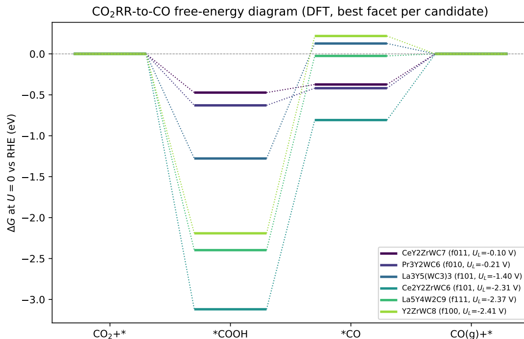
Figure 4.7: 여섯 후보의 \text{CO}_2 \rightarrow \text{CO} 전산 수소 전극(CHE) 자유에너지 다이어그램( U = 0 vs RHE, 후보별 최적 면). 낮은 과전위 후보( \text{CeY}_2\text{ZrWC}_7 , \text{Pr}_3\text{Y}_2\text{WC}_6 )는 \text{*COOH} 가 온건한 중간 상태인 반면, 나머지는 \text{*COOH} 심우물로 두 번째 환원이 강하게 흡열이다.
