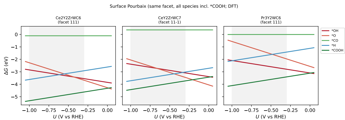
Figure 4.9: 같은-면 완전 표면 Pourbaix(DFT, *COOH 포함): *OH 면 데이터가 주 DFT와 일치하는 세 후보. 각 흡착종 \Delta G 의 전위 의존성. 작동창(음영)에서 최저 \Delta G 종이 정지상태이며, 세 후보 모두 반응 중간체 *COOH(녹색)가 우세하여 산화 피복(*OH/*O, 적색)이 지배하지 않는다.
