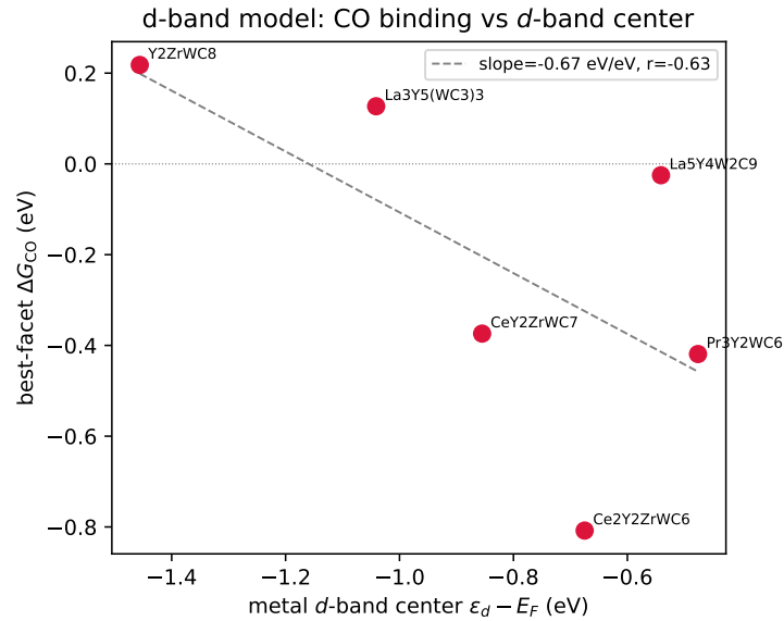
Figure 4.8: 금속 d -밴드 중심 \varepsilon_d - E_F 대 최적 면 \Delta G_{\text{CO}^*} . d -밴드가 높을수록 CO 결합이 강해지는 경향(추세선)으로 전도 특성과 흡착을 연결한다.
