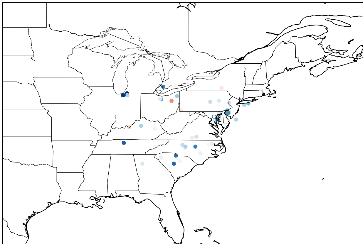
OMA (Obs - Analysis)
