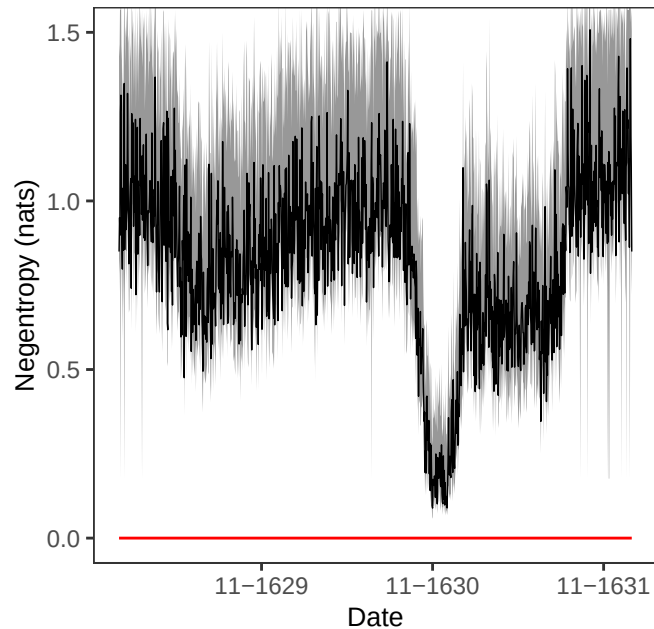
b Negentropy
