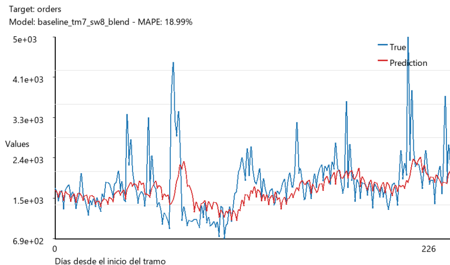
FIGURA 4.8. Predicciones vs. valores reales: Baseline .
