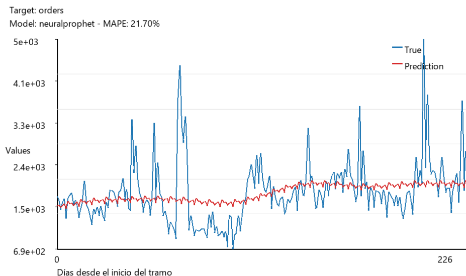
FIGURA 4.6. Predicciones vs. valores reales: NeuralProphet.
