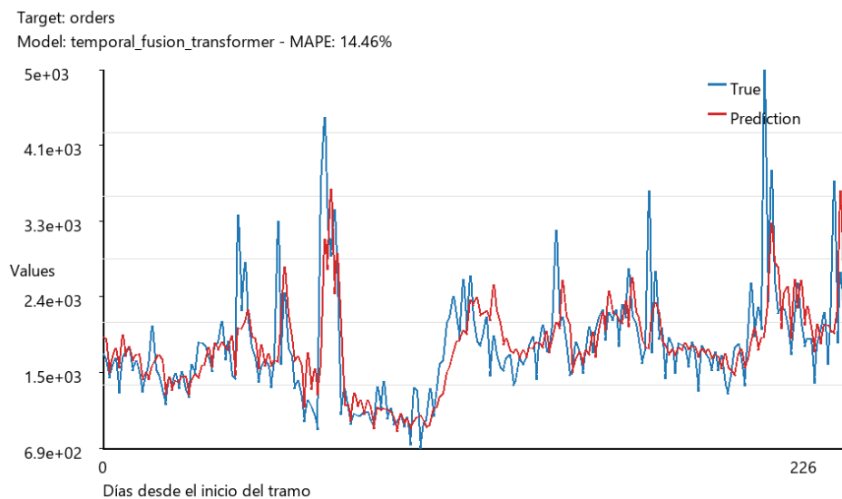
FIGURA 4.7. Predicciones vs. valores reales: TFT.
