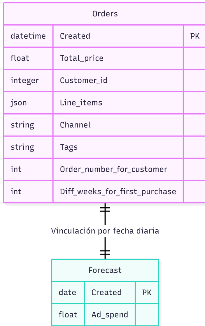
FIGURA 3.2. Diagrama entidad-relación. Muestra las dos tablas principales.
