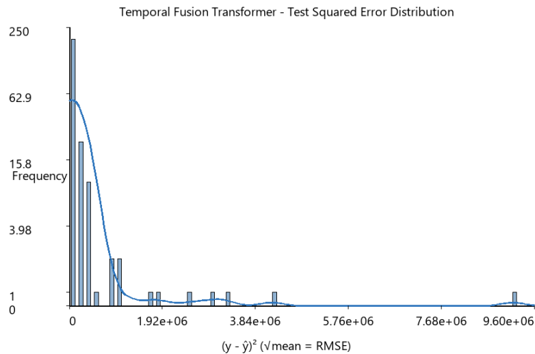
FIGURA 4.4. RMSE TFT.
