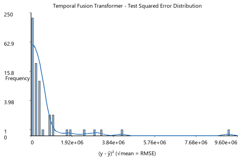
FIGURA 4.4. RMSE TFT.
