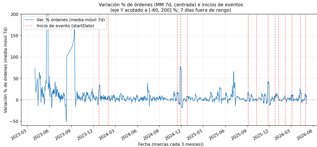
FIGURA 4.2. Variación de media movil 7 días.
