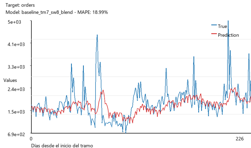
FIGURA 4.7. Comparativa de predicciones vs. valores reales: Mezcla lineal frente a Baseline.
