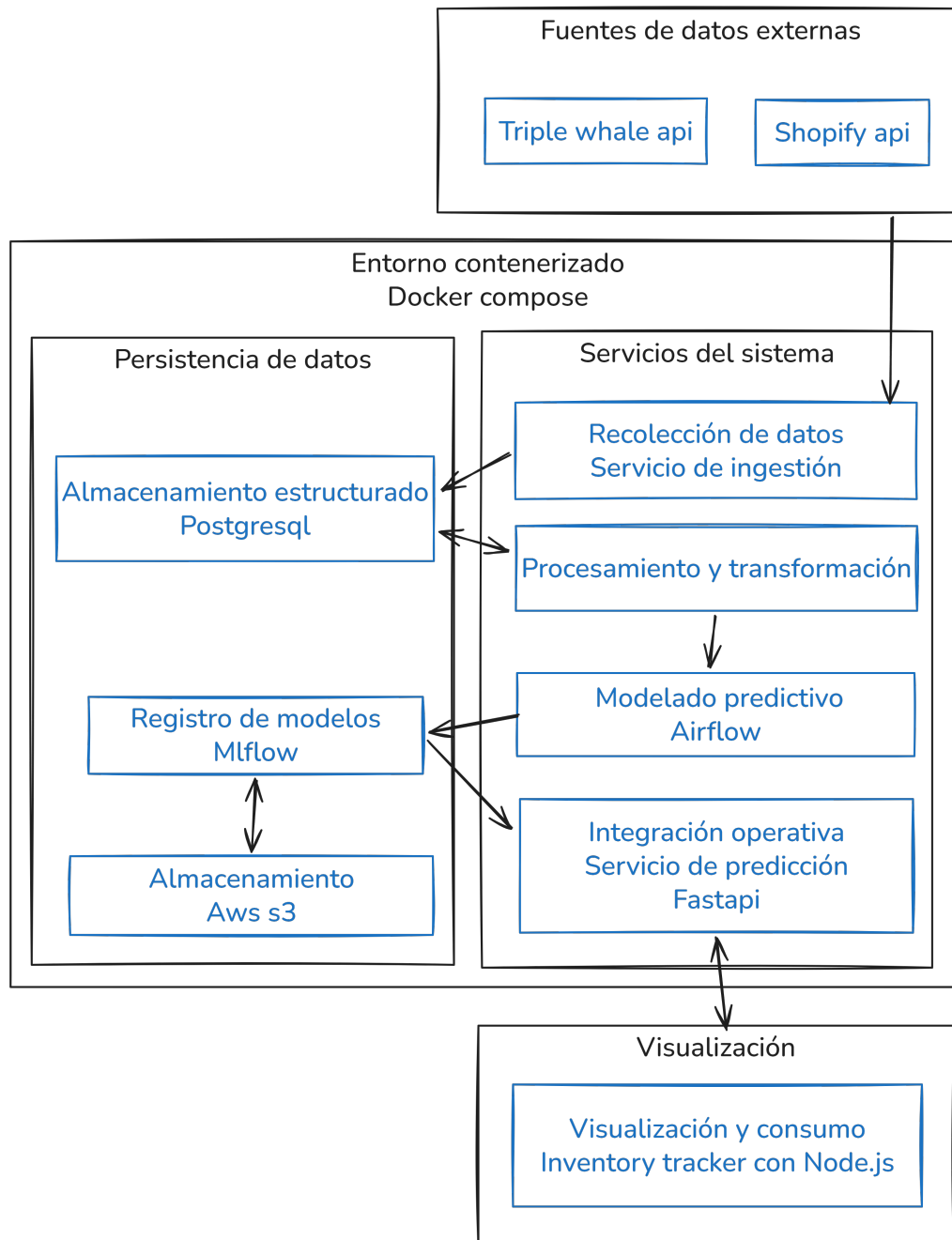
FIGURA 3.1. Diagrama de arquitectura del sistema.
