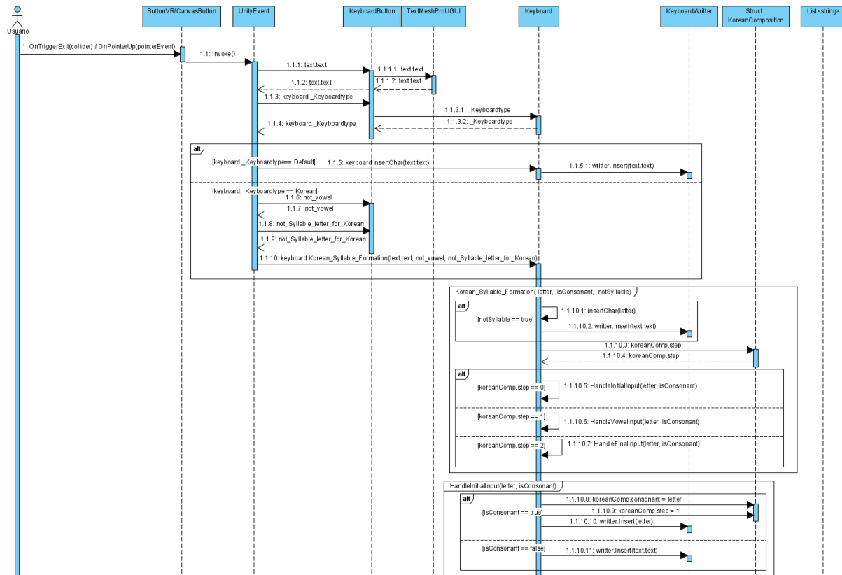
Figura 5.11: Primer fragmento del diagrama de secuencia que muestra el proceso para añadir un carácter
