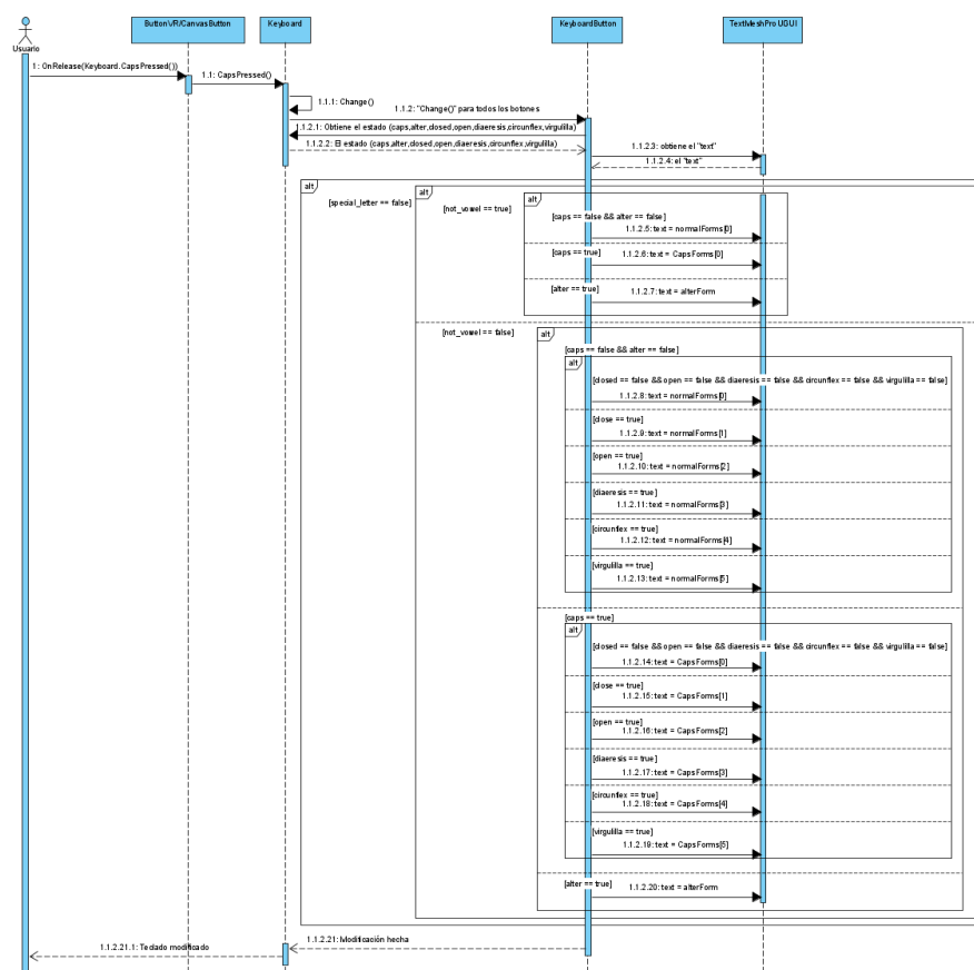
Figura 4.6: Diagrama de secuencia de la modificación de las letras de un teclado
