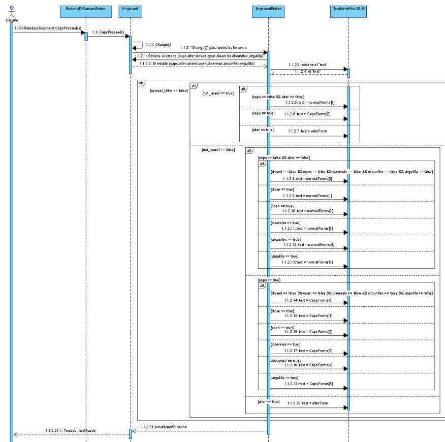
Figura 4.5: Diagrama de secuencia de la modificación de las letras de un teclado
