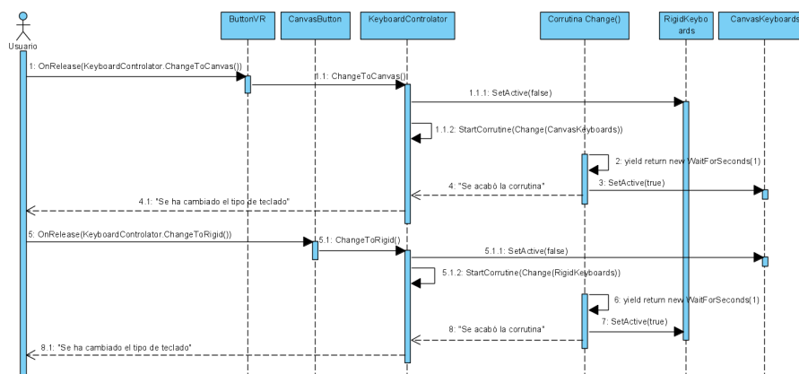
Figura 4.4: Diagrama de secuencia para el cambio de tipo de teclado
