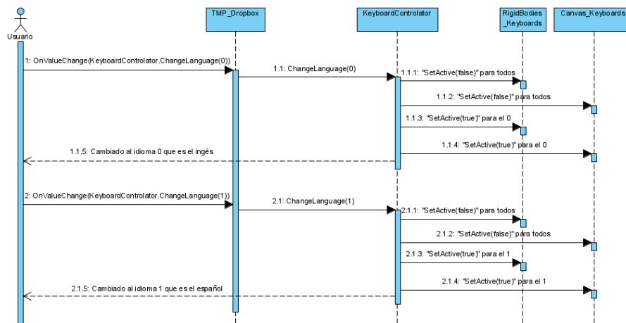
Figura 4.3: Diagrama de secuencia para cambiar de idiomas
