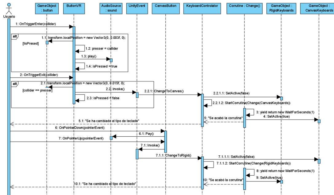
Figura 5.3: Diagrama de secuencia para el cambio de tipo de teclado
