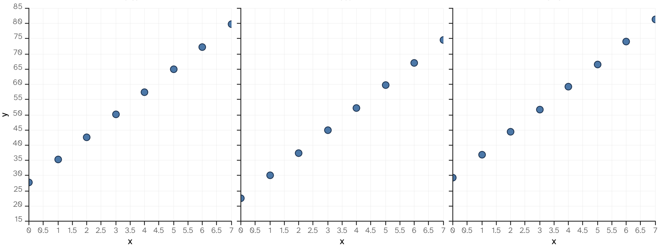
Boreal
