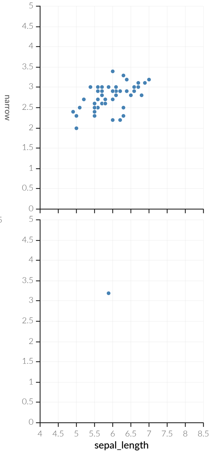
Iris-versicolor
