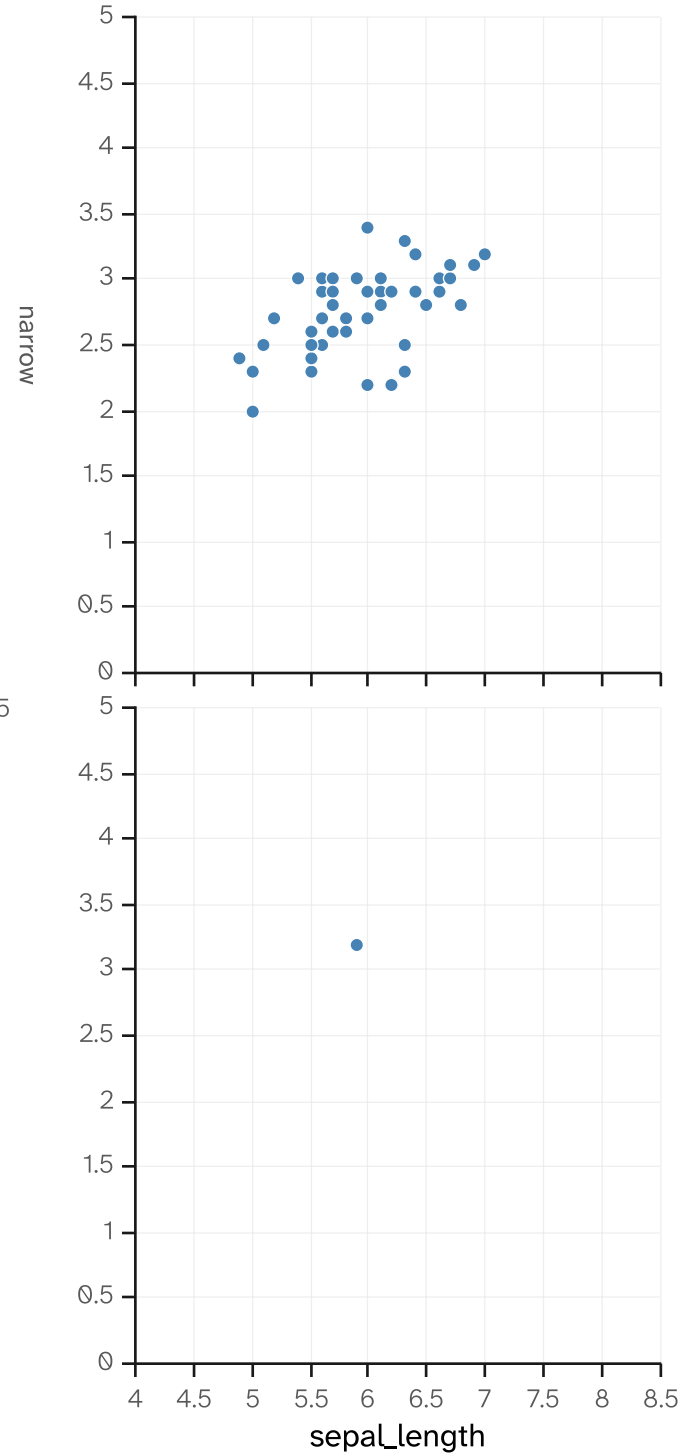
Iris-versicolor
