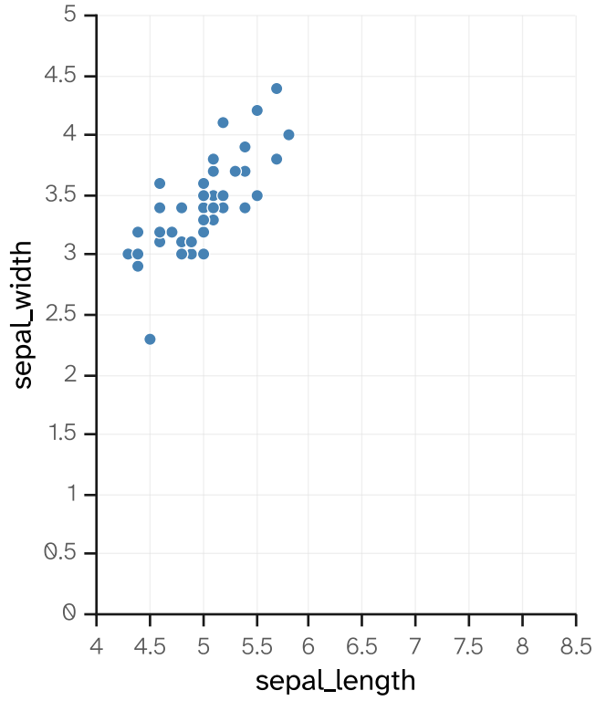
Iris-setosa
