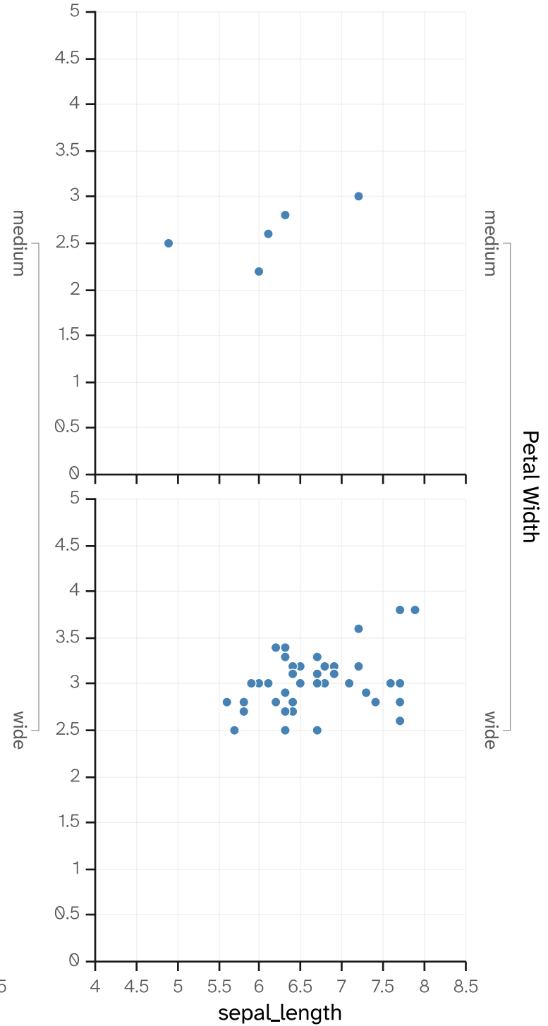
Iris-virginica
