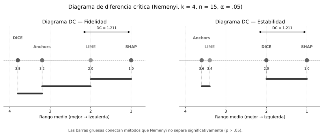
Figura 9. Diagrama de diferencia crítica de Nemenyi para fidelidad y estabilidad. Fuente: elaboración propia a partir de las tablas de rangos y comparaciones de Nemenyi de EXP2.
