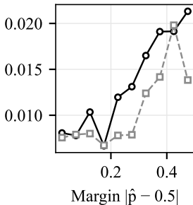
LIME
