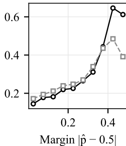
DiCE
