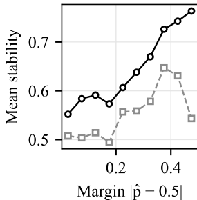
SHAP
