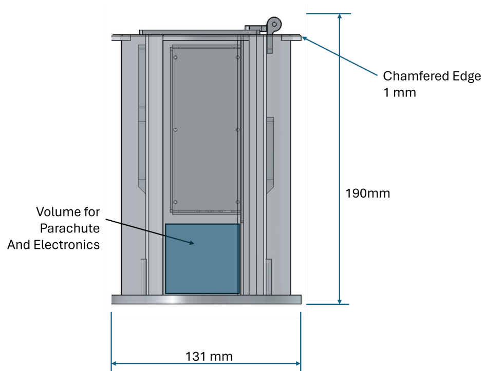
Container Dimensions
