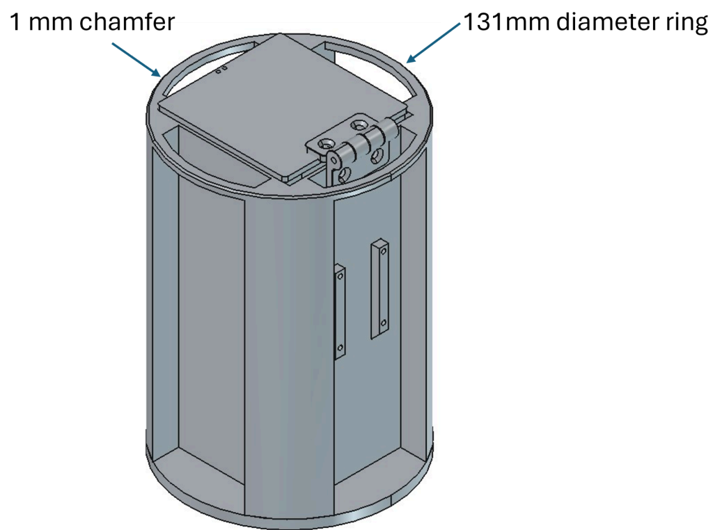
Container Top Dimensions
