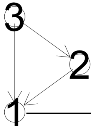
True DAG
