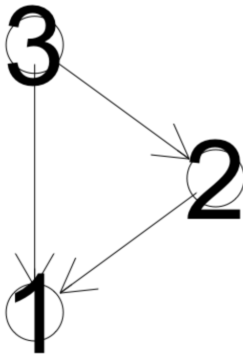
True DAG
