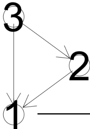
True DAG
