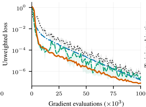
PirateNet: KdV
