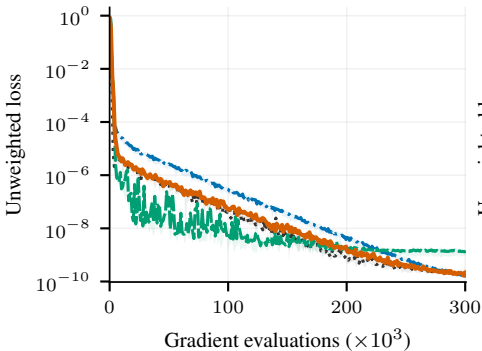
PirateNet: Allen-Cahn
