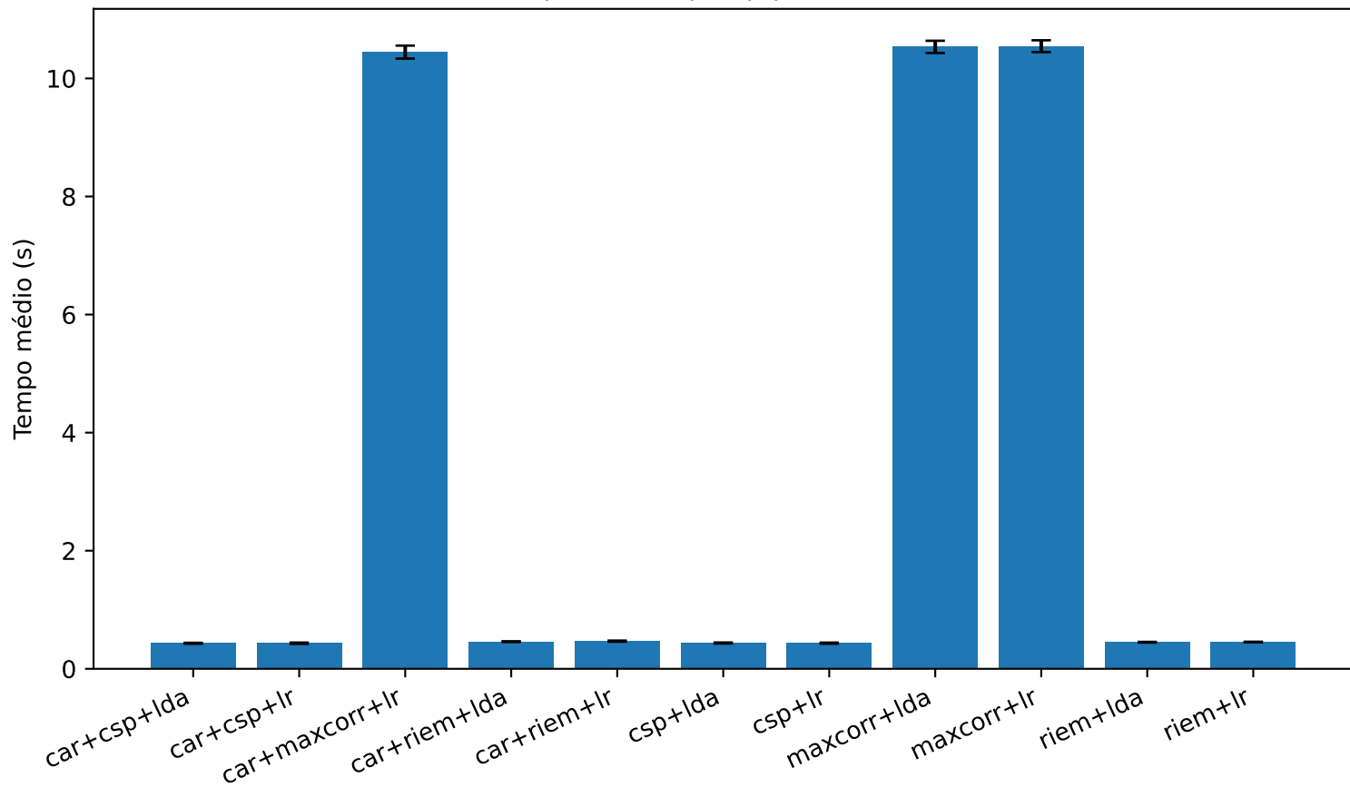
Tempo médio por pipeline ( \pm EP)
