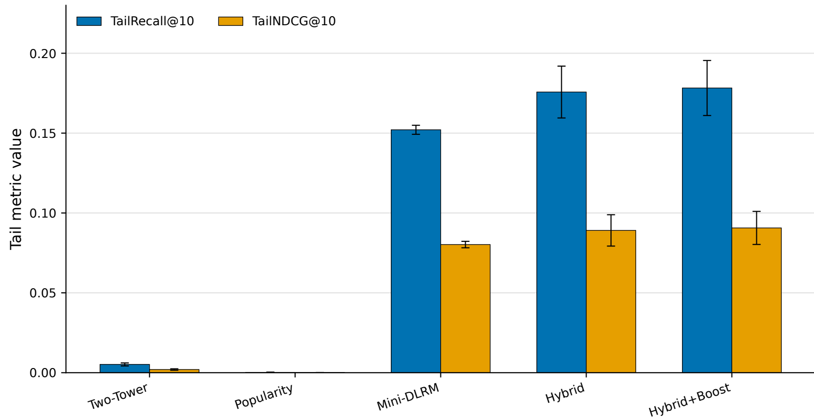
Tail-item relevance
