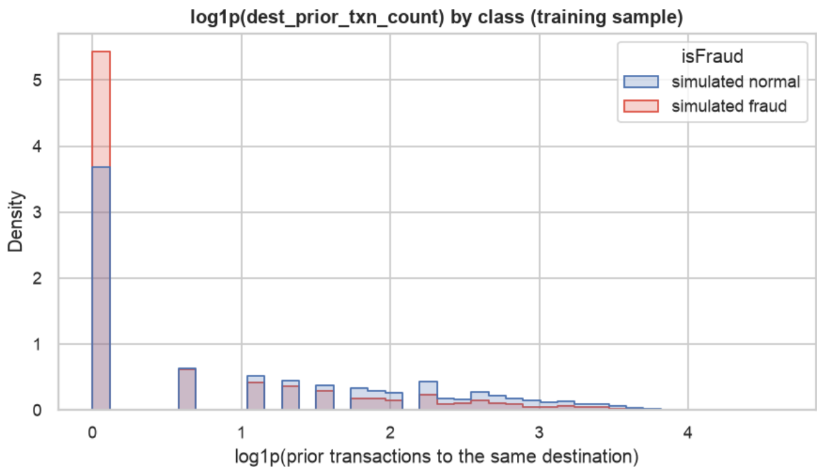
Figure: eda_11_dest_prior_count.png
