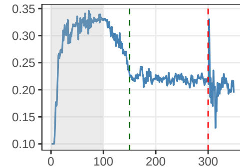
-L_\psi(x)
