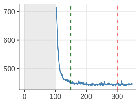
-L_\psi(x)
