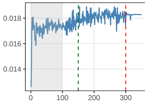
\omega_{k_e}
