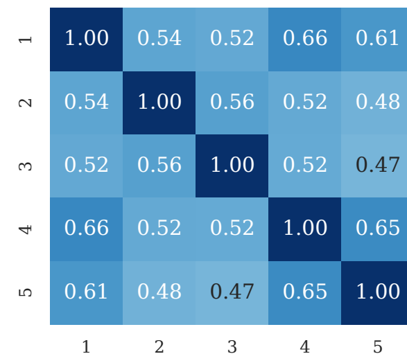
GPT-4o-mini
