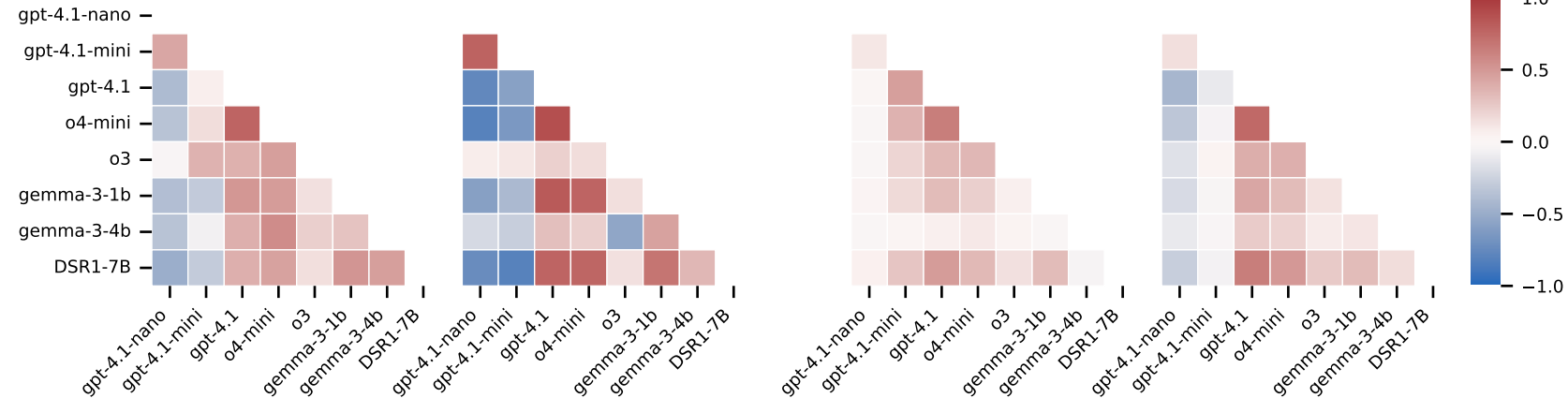
101-200 productions
