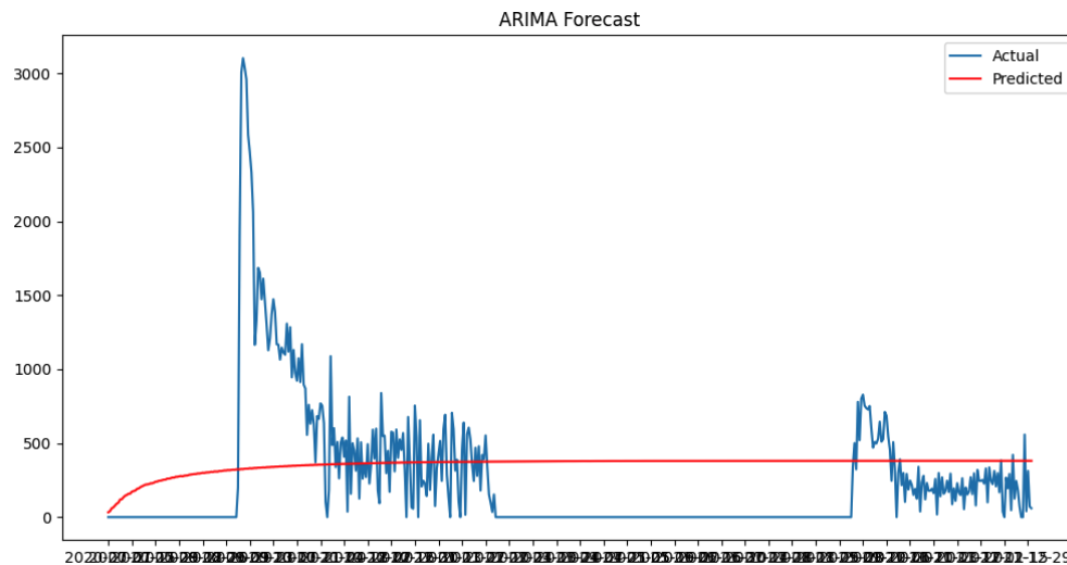
Figure 9: ARIMA: Predicción de ambas temporadas — Valores reales (azul) contra valores predichos (rojo)
