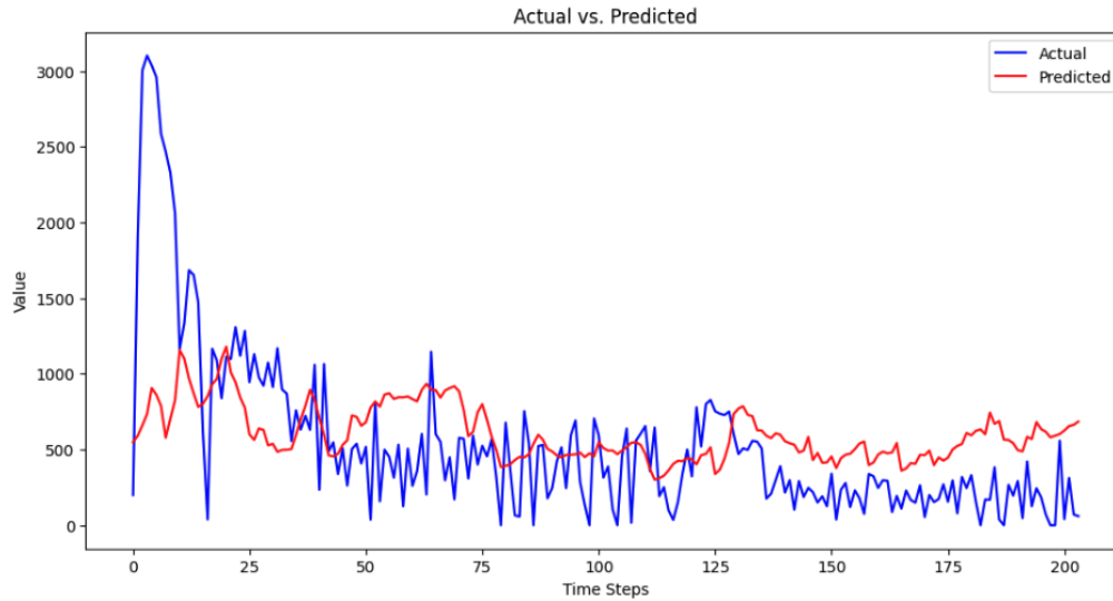
Figure 15: XGBoost + LSTM — Predicción temporadas 2020-2021 y 2021-2022: Valores reales (azul) contra valores predichos (rojo). Nota: Aquí no aparecen las fechas consideradas como veda (periodo entre temporadas)
