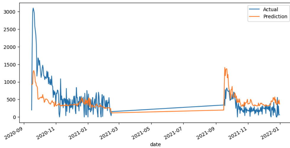
Figure 11: XGBoost: Predicción de ambas temporadas — Valores reales (azul) contra valores predichos (naranja)
