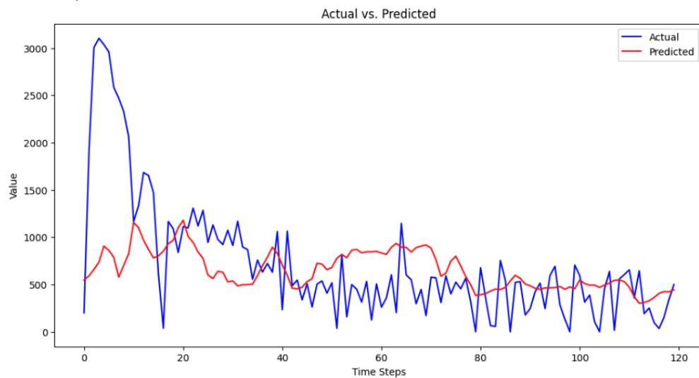
Figure 13: XGBoost + LSTM — Predicción temporada 2020-2021: Valores reales (azul) contra valores predichos (rojo)
