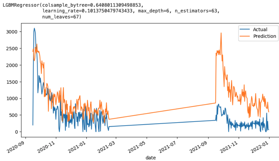
Figure 12: LGBM: Predicción de ambas temporadas — Valores reales (azul) contra valores predichos (naranja)
