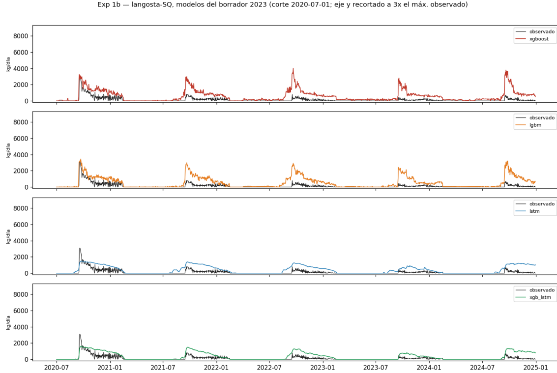
Figure 8: Langosta \times San Quintín en el corte 01-julio-2020: observado (negro) contra los cuatro modelos de aprendizaje del borrador. Los cuatro sobre-predicen las temporadas posteriores al bache; la LSTM y el ensamble lo hacen menos porque aplanan la serie en una meseta suave, no porque sigan mejor su forma —de ahí su menor MAE con una correlación equivalente. Eje y recortado a 3\times el máximo observado.
