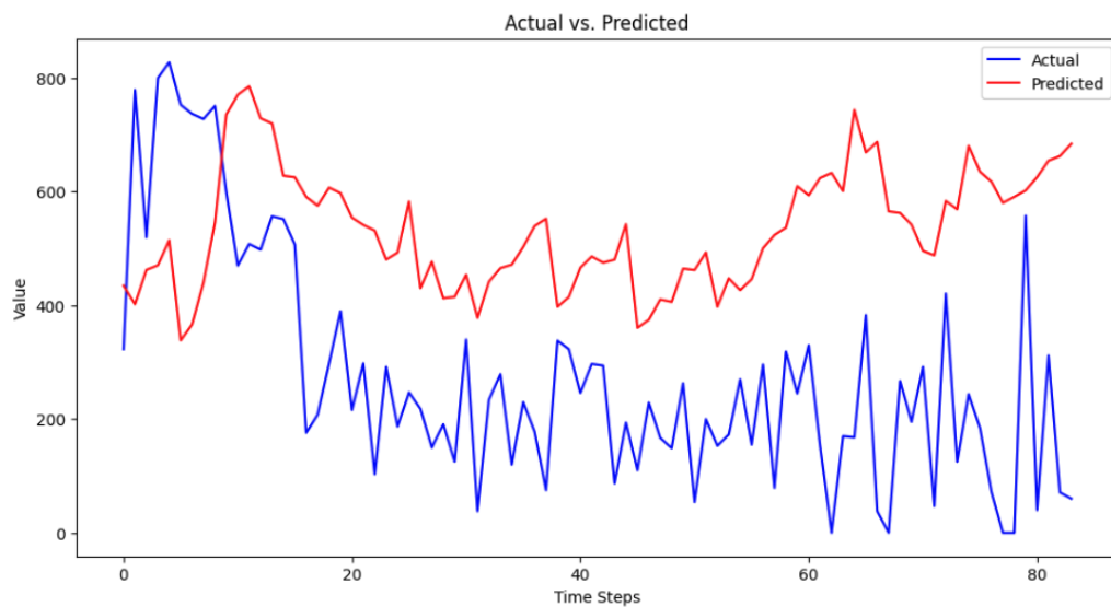
Figure 14: XGBoost + LSTM — Predicción temporada 2021-2022: Valores reales (azul) contra valores predichos (rojo)
